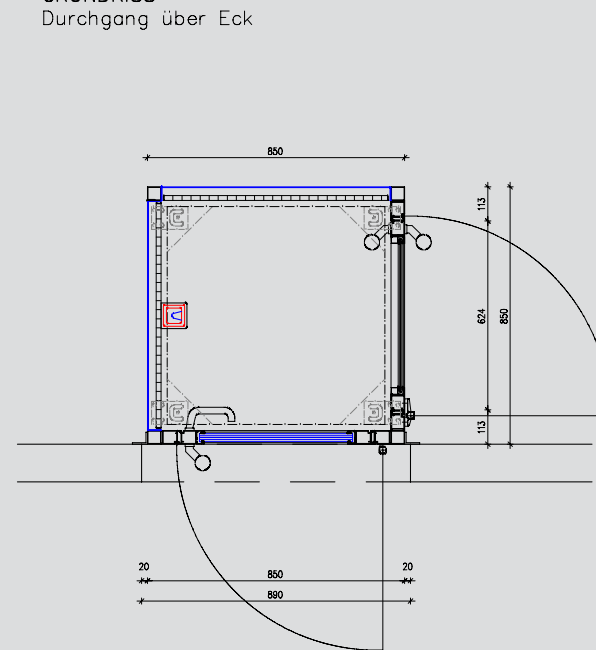
GRUNDRISSE Durchgang über Eck
