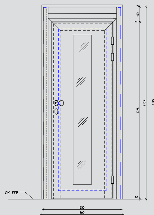
ANSICHT AUSSEN TÜR
