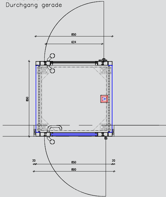
GRUNDRISSE Durchgang gerade
